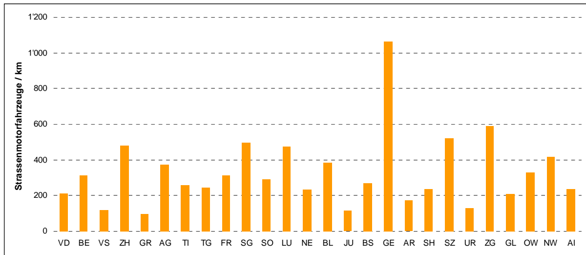
Abbildung 3: Motorfahrzeuge pro km Kantonsstrasse nach Kantonen
