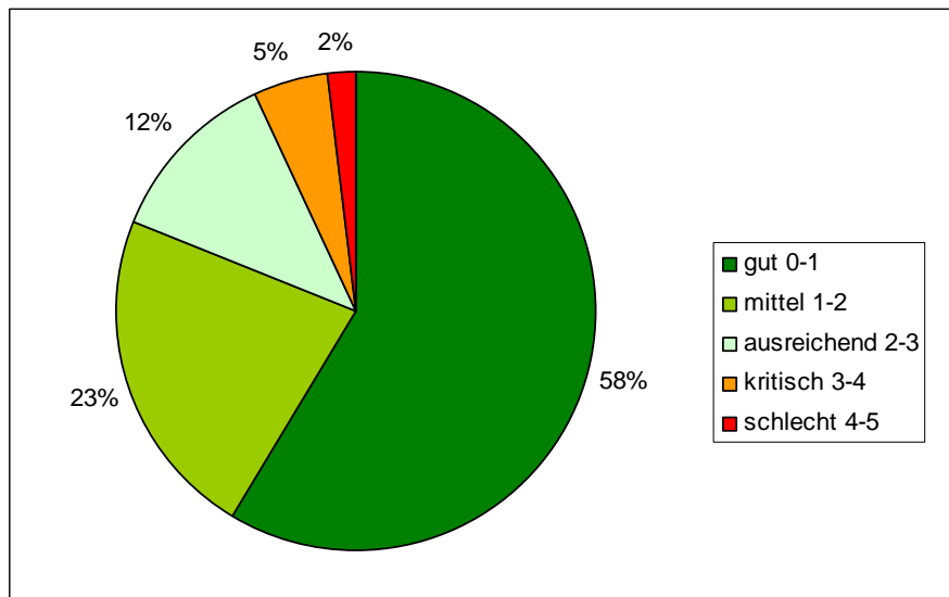
Abbildung 8: Ebenheit in Querrichtung I 3 der Kantonsstrassen
