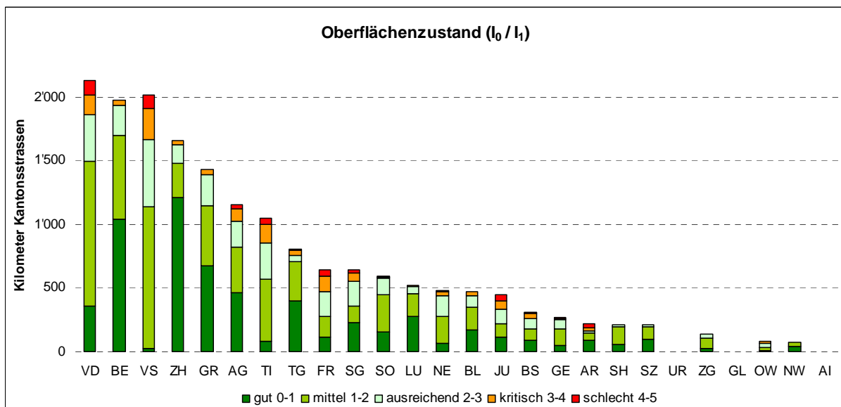
Abbildung 6: Oberflächenzustand des Kantonsstrassennetzes nach Kantonen in km
