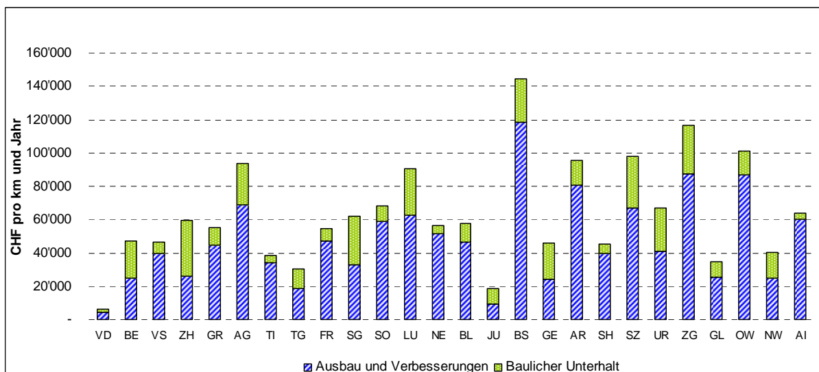
Abbildung 13: Ausgaben für Verbesserungen und Ausbau sowie baulichen Unterhalt pro km nach Kantonen
