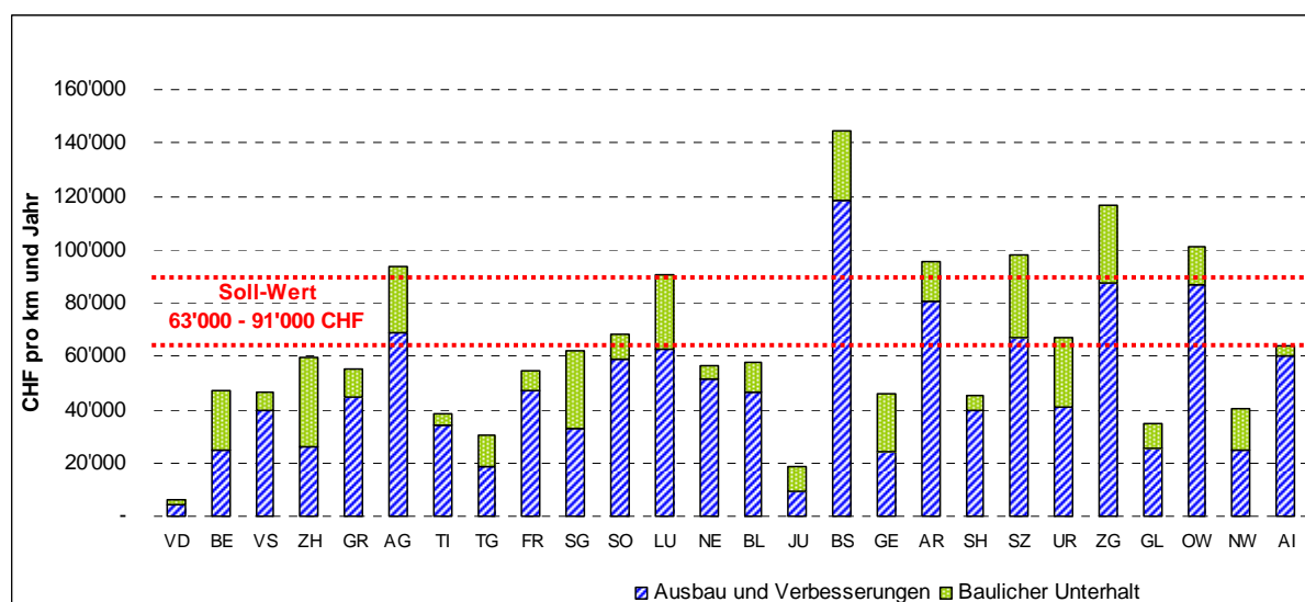
Abbildung 15: Soll-Ist-Vergleich betreffend Substanzerhaltung nach Kantonen
