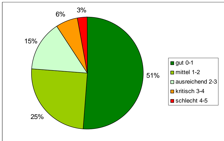
Abbildung 7: Ebenheit in Längsrichtung I 2 der Kantonsstrassen
