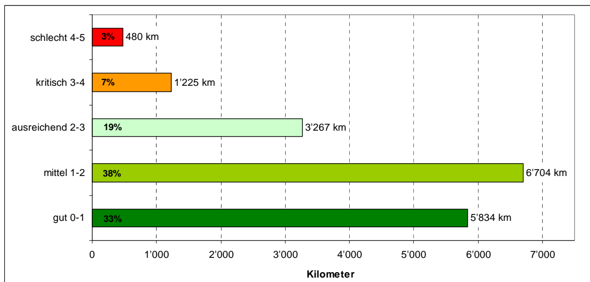
Abbildung 4: Oberflächenzustand aller Kantonsstrassen der Schweiz
