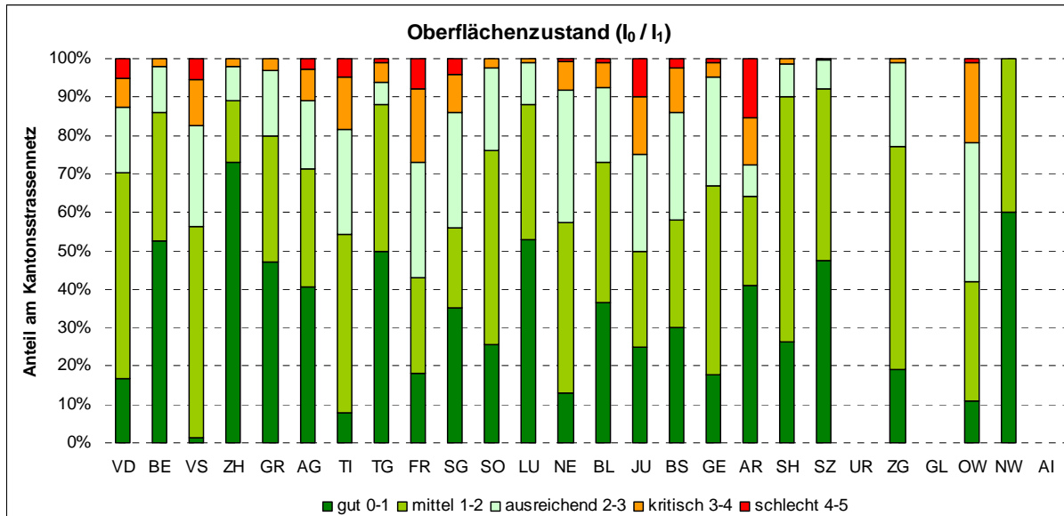
Abbildung 5: Oberflächenzustand des Kantonsstrassennetzes nach Kantonen in %
